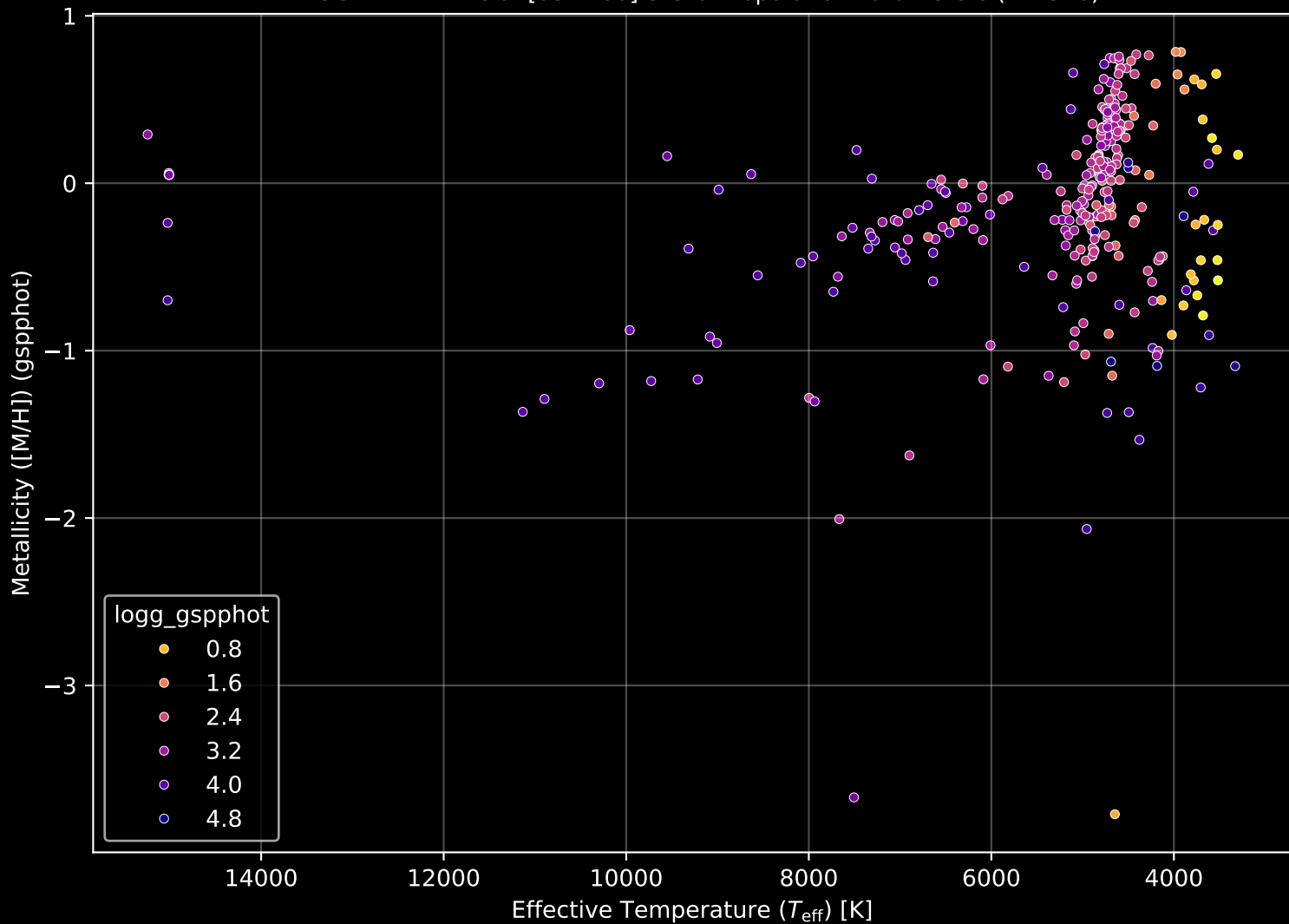
APOGEE DR17 Field: [034+00] Stellar Population Parameters (n= 320)
